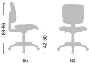
XA10 - XA20 Sedia ergonomica bassa senza braccioli mov. 10X. Low ergonomic chair mov. 10X.
