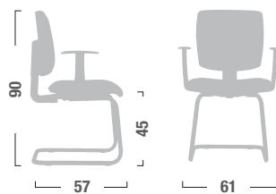
XA18 - XA28 Sedia fissa con braccioli. Fixed armchair.
