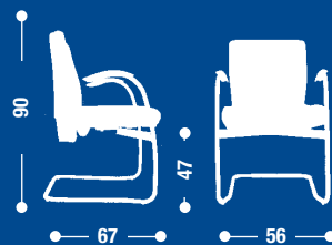
TK36 Sedia fissa con braccioli. Fixed armchair.
