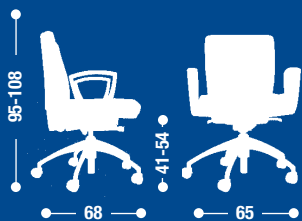
TK33 Poltrona ergonomica alta con oscillante mov. 1. High ergonomic armchair w/tilting mov. 1.
