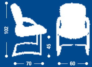
RP 18 Poltrona attesa fissa con braccioli Fixed armchair
