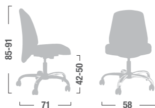
L44C Poltrona girevole senza braccioli mov. 19. Swivel chair mov. 19.
