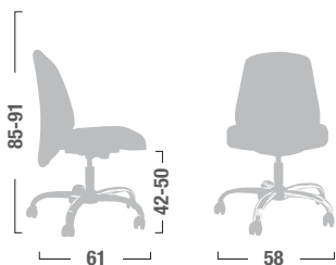
L44A Poltrona girevole senza braccioli. Swivel chair.
