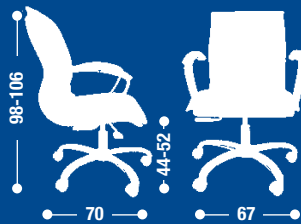
GL24 Poltrona direzionale con braccioli senza oscillante. Directional armchair without tilting.
