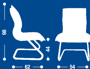
GL27 Poltrona attesa fissa senza braccioli. Fixed chair.
