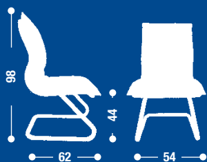
GL17 Poltrona attesa fissa senza braccioli. Fixed chair.
