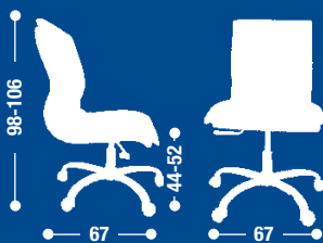
GL25 Poltrona visitatore girevole senza braccioli. Swivelling chair.
