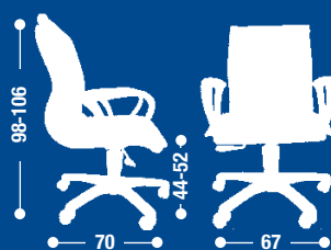
GL14 Poltrona direzionale con braccioli senza oscillante. Directional armchair without tilting.
