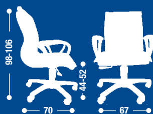
GL13 Poltrona direzionale con braccioli e oscillante mov. 3. Directional armchair with mov. 3 tilting.
