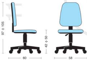
BS 14 BS 24 Sedia dattilo ergonomica alta senza braccioli mov. 10-15
