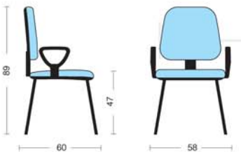
BS 18 Sedia fissa con braccioli Fixed armchair
